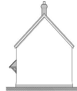
FLANK ELEVATION
